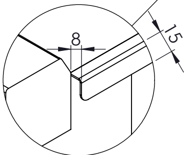
DETTAGLIO SCALA 1 : 2
